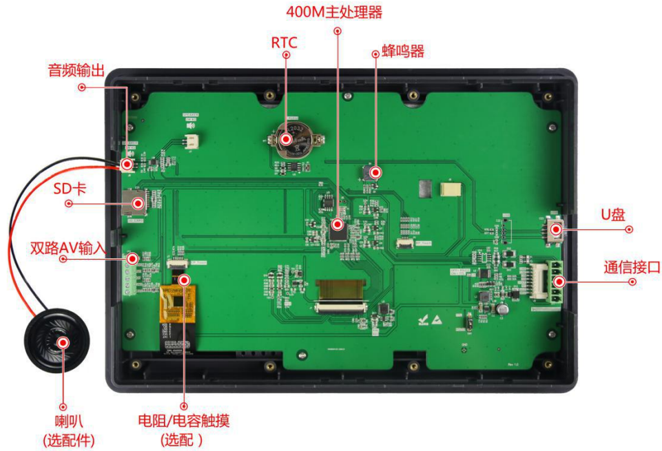
图 1-3 硬件配置图
