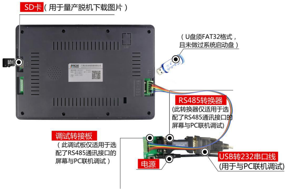
图 1-5 RS485 调试工具图
