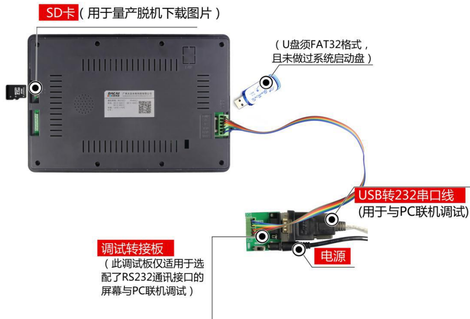
图 1-4 RS232 调试工具图
