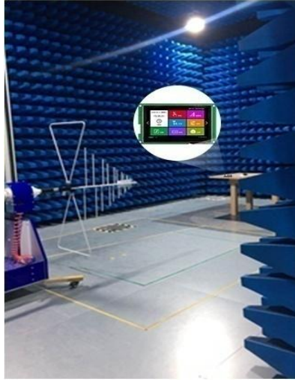
图 6-5 辐射测试图
