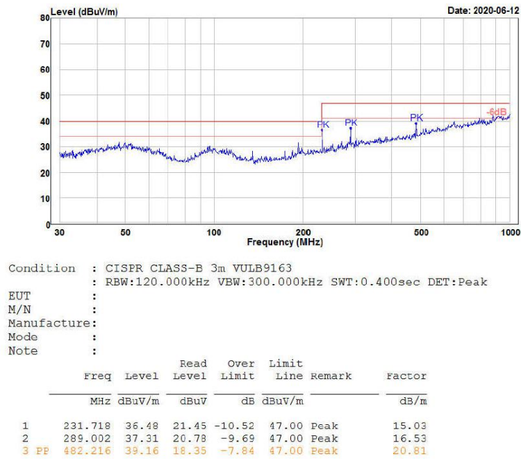
图 6-6 辐射测试水平方向
